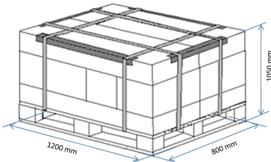
Abbildung 2: Standardpalettenmaß
